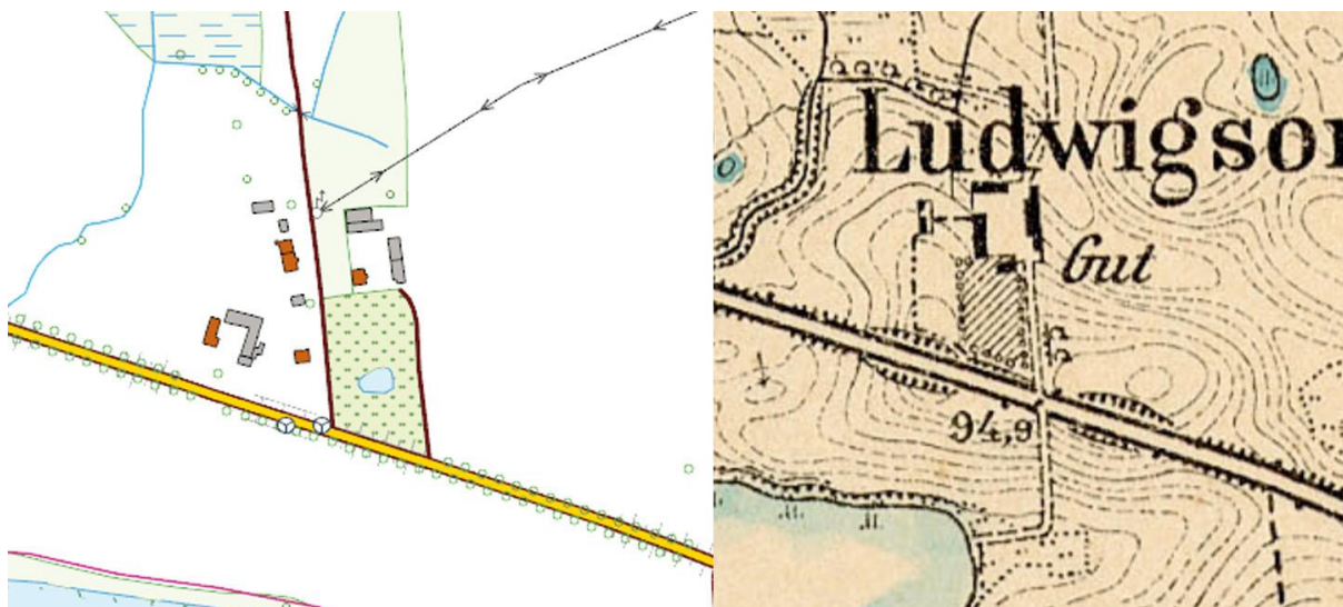
Ryc. 5. Ludwichowo. Zespół podworski (opracowanie własne: mapa 1. Podkład www.geoportal.gov.pl ; mapa 2. Mapa Messtischblatt, 1910 r.).
