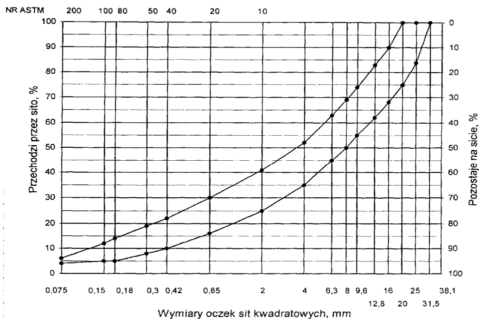
Rys. 12. Krzywe graniczne uziarnienia mieszanki mineralnej BA od 0 do 20 mm do warstwy wiążącej, wyrównawczej i wzmacniającej
