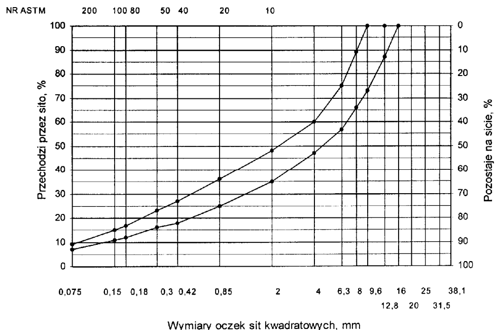
Rys. 7. Krzywe graniczne
