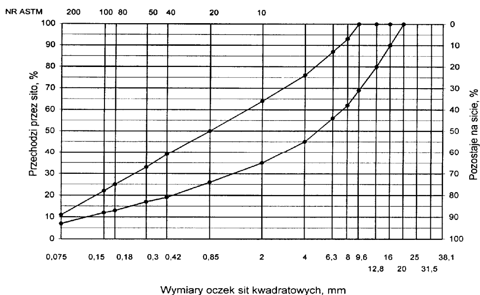
Rys. 2. Krzywe graniczne uziarnieni a mieszanki mineralnej BA od 0 do 16mm, od 0 do 12,8 mm do warstwy ścieralnej nawierzchni drogi o obciążeniu u ruchem KR1 lub KR2
