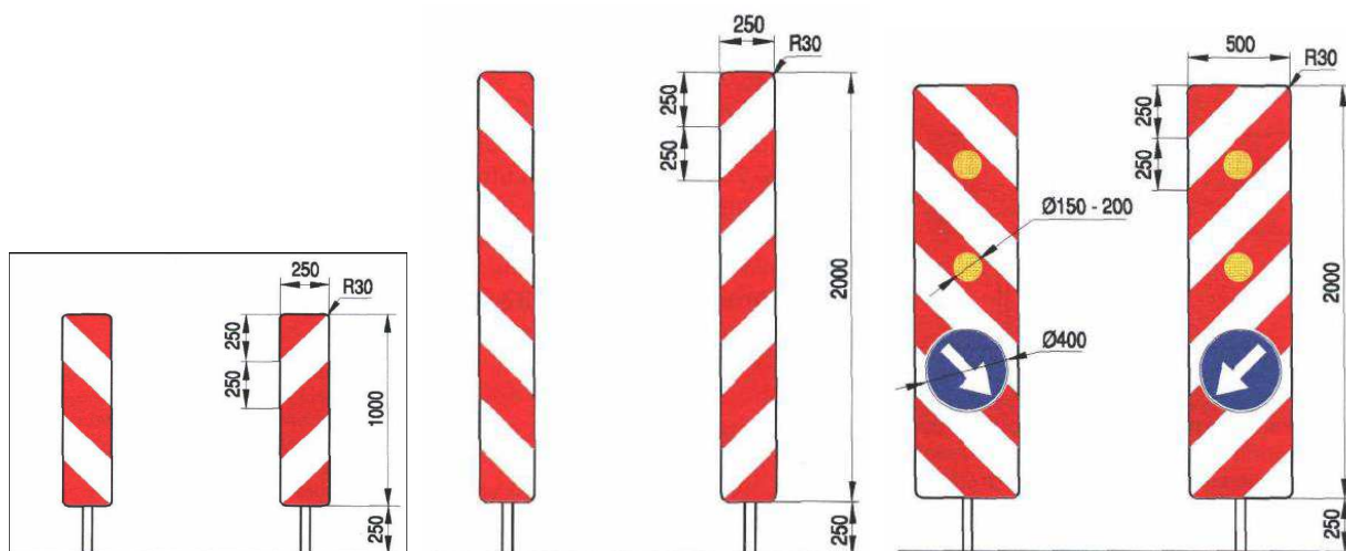
a) U-21a b) U-21b
