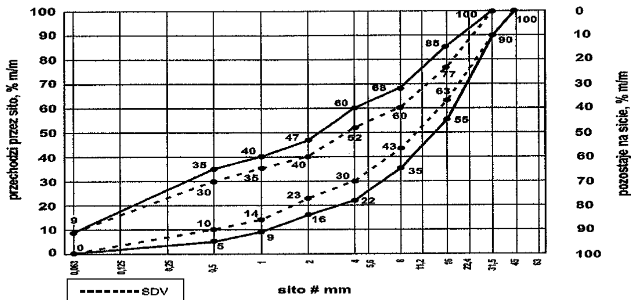
Rys. 1. Krzywe graniczne uziarnienia mieszanki kruszywa niezwiązanego 0/31,5 mm do warstw podbudowy zasadniczej Oprócz wymagań podanych na rys. 1, wymaga się aby 90% uziarnień mieszanek zbadanych w ramach ZKP w okresie 6 miesięcy spełniało wymagania kategorii podanych w tablicach 2 i 3, aby zapewnić jednorodność i ciągłość uziarnienia mieszanek.
