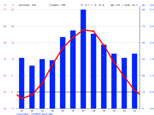
Wykres 5. Klimatogram Miasta i Gminy Łasin
